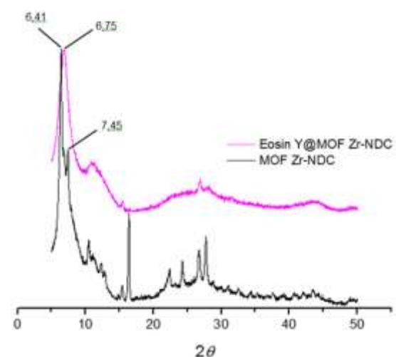
Gambar 1. Hasil analisis PXRD MOF Zr-NDC.
