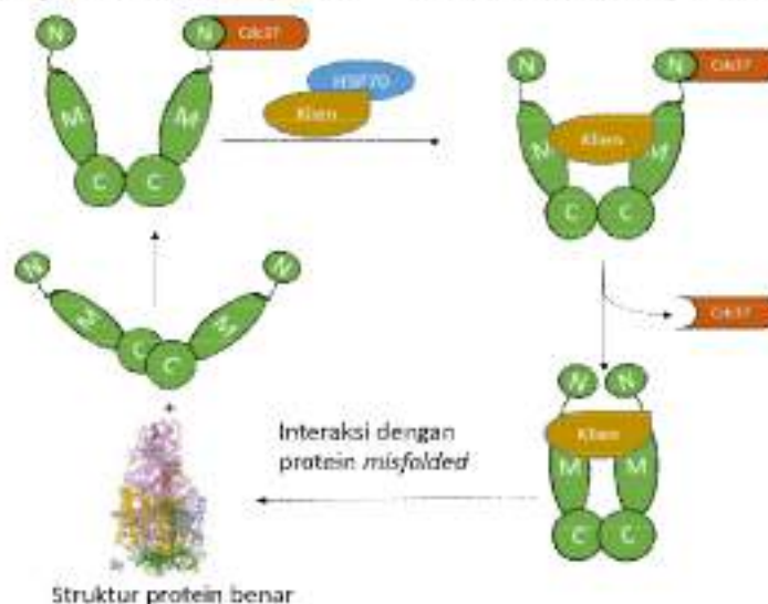
Gambar 2. Mekanisme kerja HSP90
