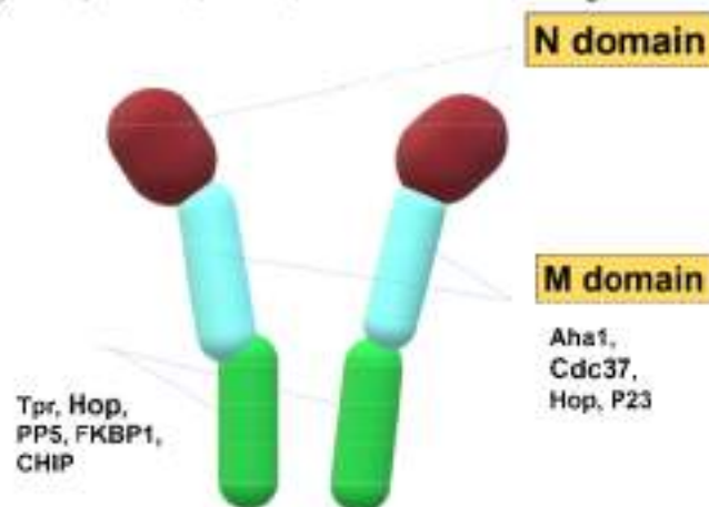
Gambar 3. Struktur HSP90 dan interaksinya dengan beberapa protein
