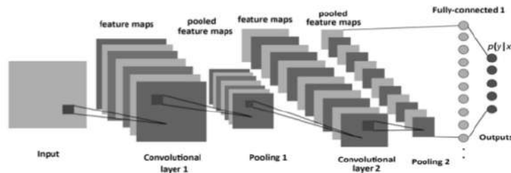
Gambar 2. Arsitektur dasar CNN [18]
