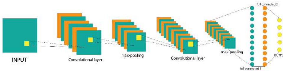
Gambar 6. Ilustrasi desain arsitektur LeNet
