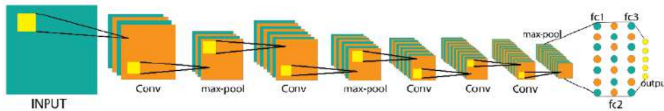
Gambar 7. Ilustrasi desain arsitektur AlexNet
