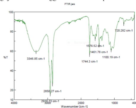
Gambar 5 Karakteristik FT-IR
