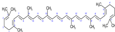
Gambar 1. Struktur Likopen
