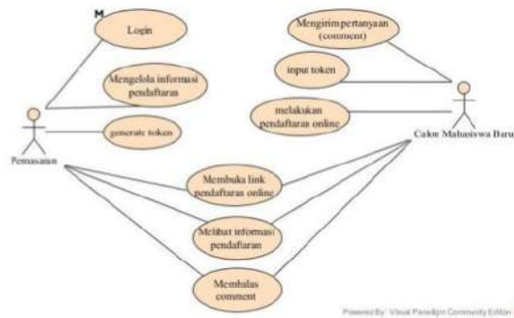
Gambar 3. Use Case Diagram Modul Informasi Pendaftaran
