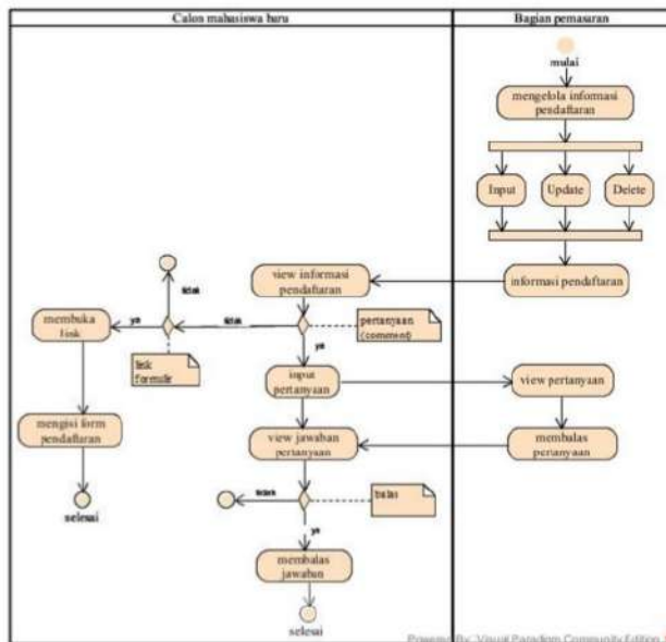
Gambar 4. Activity Diagram Modul Informasi Pendaftaran
