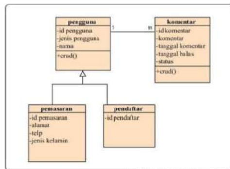
Gambar 5. Class Diagram Modul Informasi Pendaftaran
