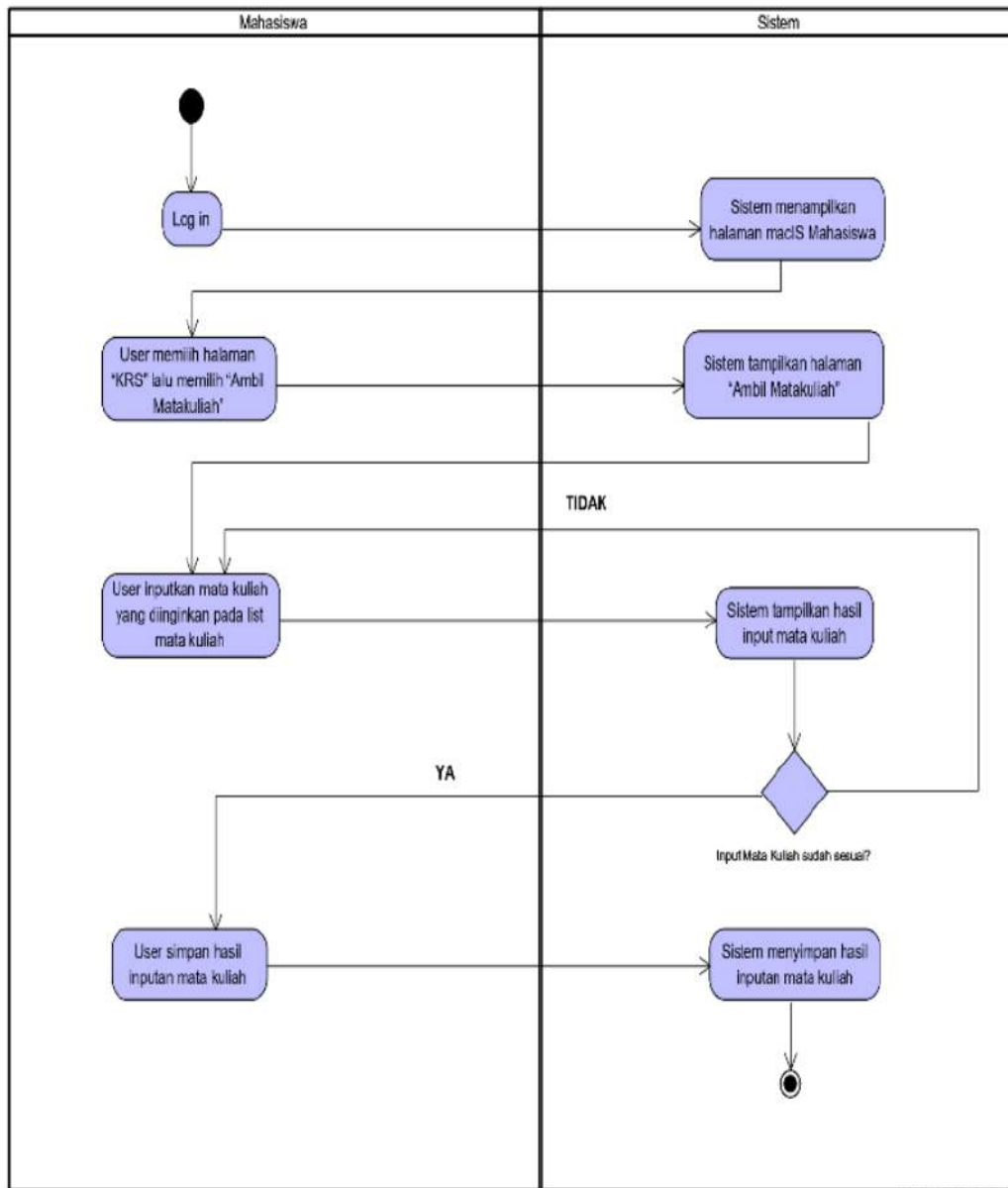
Gambar 4 Diagram Aktivitas KRS – Ambil Matakuliah
