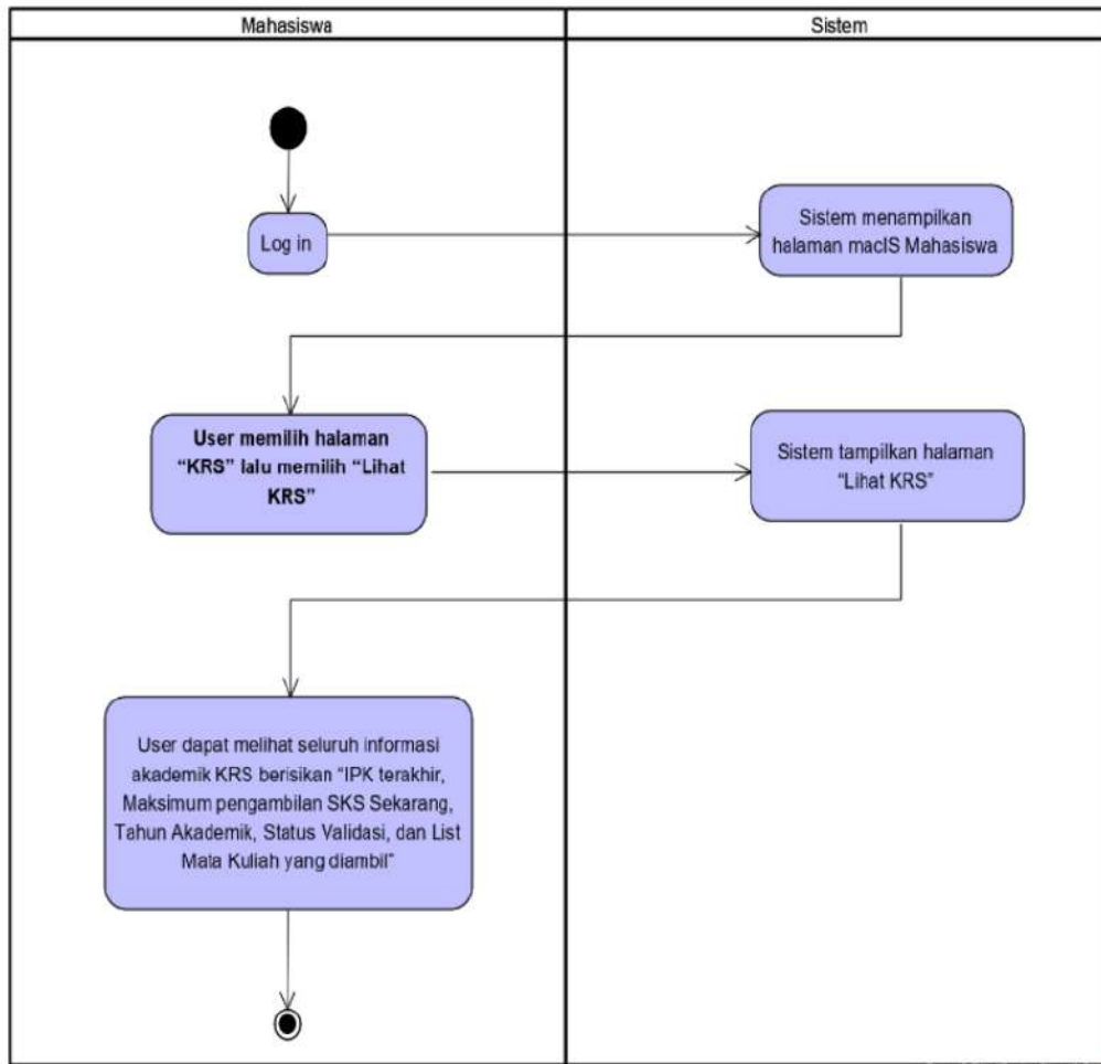
Gambar 5 Diagram Aktivitas KRS – Lihat KRS
