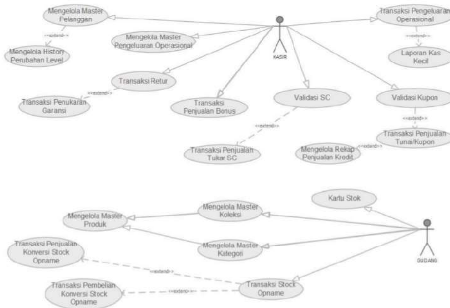
Gambar 6. Diagram Use Case untuk Aktor Gudang & Kasir
