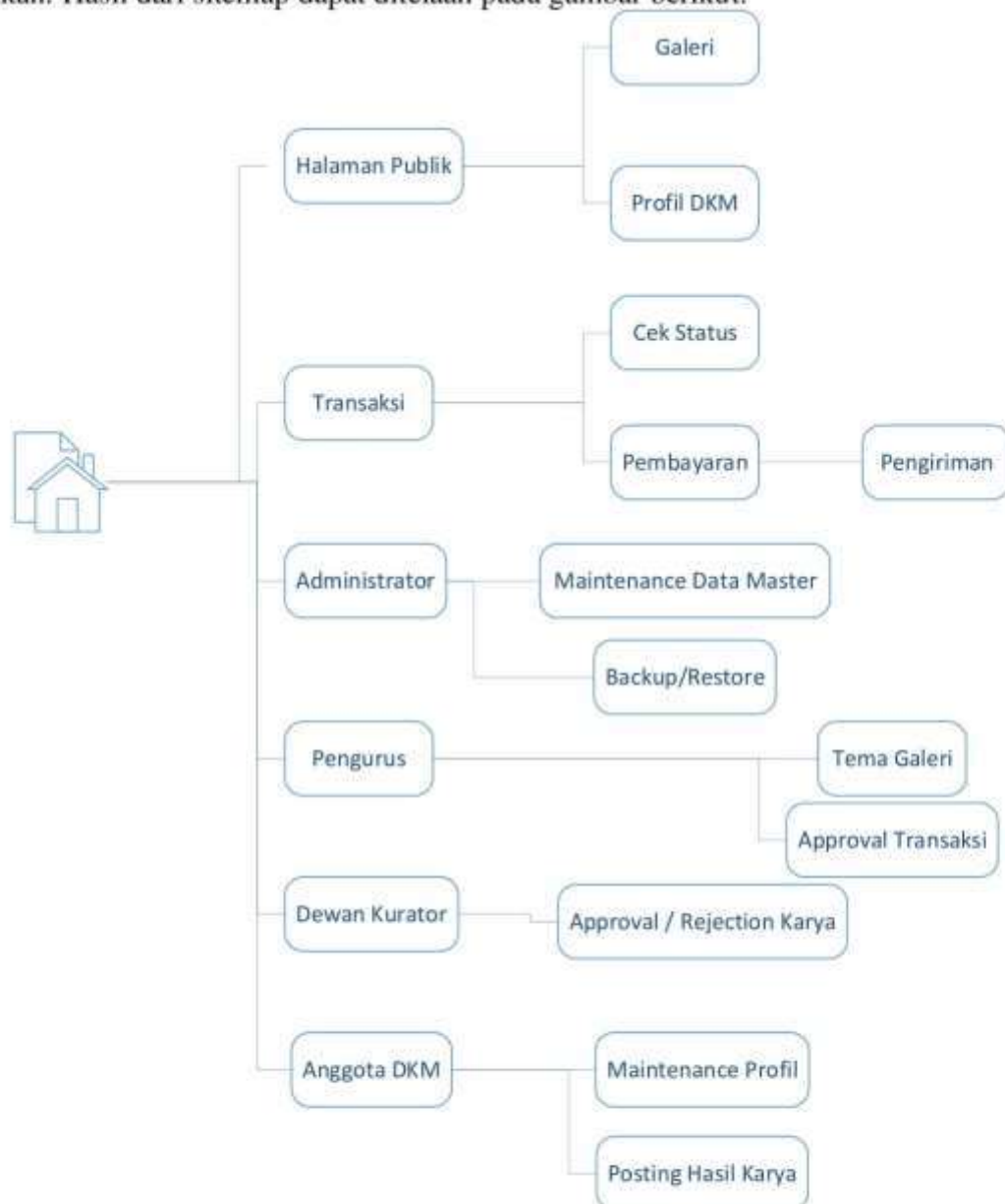
Gambar 3. Sitemap Awal
