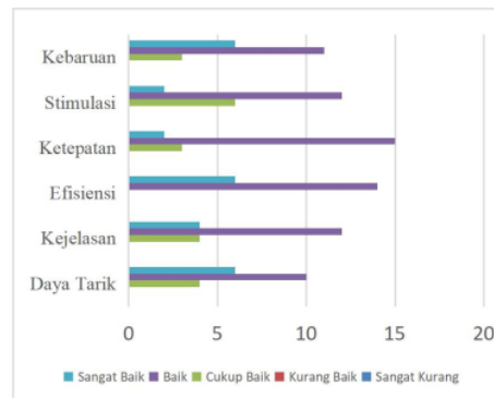
Gambar 16. Hasil Angket Penilaian UI/UX
