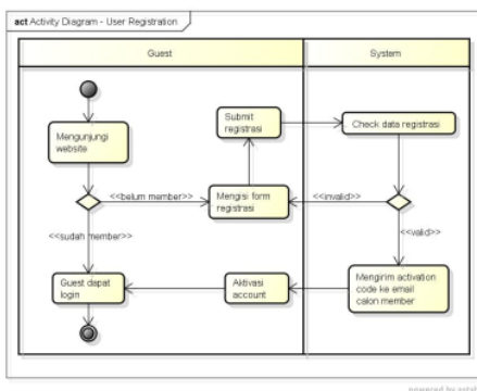
Gambar 2. Detil Proses Registrasi User
