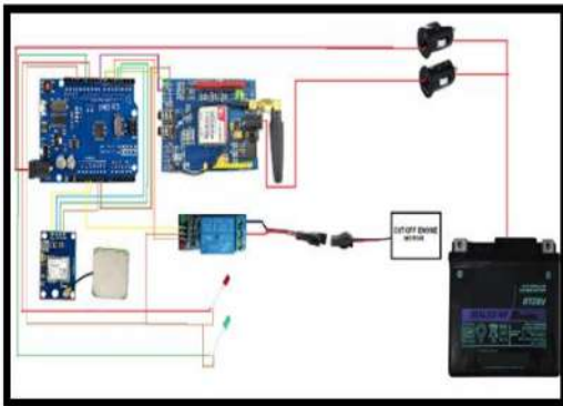
Gambar 11 Rangkaian keseluruhan prototipe
