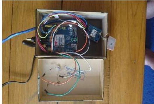
Gambar 12 Rangkaian Perangkat Keras
