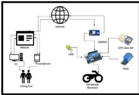
Gambar 9 Topologi Sistem Monitoring kendaraan bermotor
