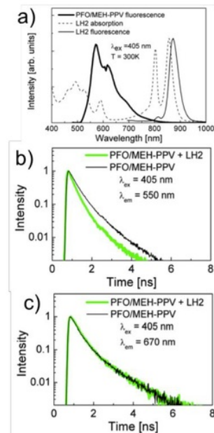
Gambar 4. Spektra absorpsi dan fluoresensi LH2 dan polimer PFO/MEH-PPV (a), dan pengukuran peluruhan fluoresensi pada sistem kombinasi LH2-PFO/MEH-PPV [9].
