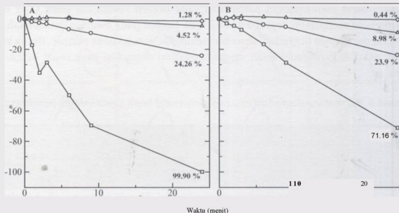
Gambar 5. Grafik kinetika degradasi ekstrak kasar karotenoid buah kelapa sawit segar (A) dan buah sawit yang direbus (B) yang dipanaskan pada suhu kontrol (25°C) ( ○ ), 50°C ( ⊗ ), 65°C ( ◊ ) dan 90°C ( □ ) pada panjang gelombang deteksi 450 nm.
