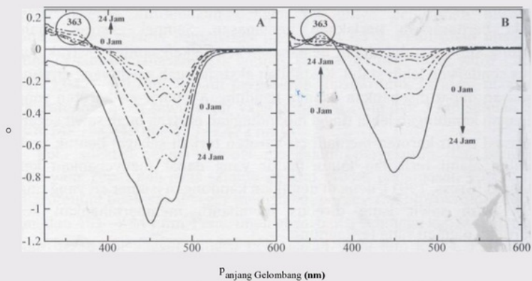
Gambar 6. Absorpsi spektra ( Different Absorbition Spectra ) ekstrak karotenoid buah sawit segar (A) dan rebus (B) dengan lama perlakuan pemanasan 1 jam ( - - ), 2 jam ( ..... ), 3 jam ( ———— ), 6 jam ( - - - - - ), 9 jam ( ———— ), dan 24 jam ( ———— ).
