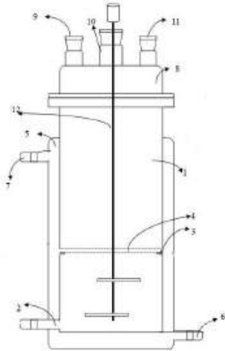
Gambar 1. Reaktor tampak depan
