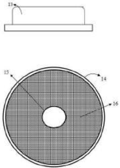
Gambar 2. Tutup reaktor tanpa pengaduk dan penyaring tampak atas
