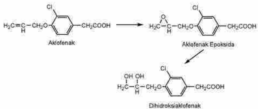
Gambar 47. Biotransformasi Karbamazepin dan Aklofenak
