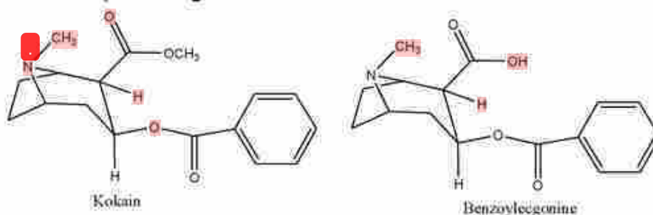
Gambar 24. Hidrolisis Kokain menjadi Benzoylecgonine
