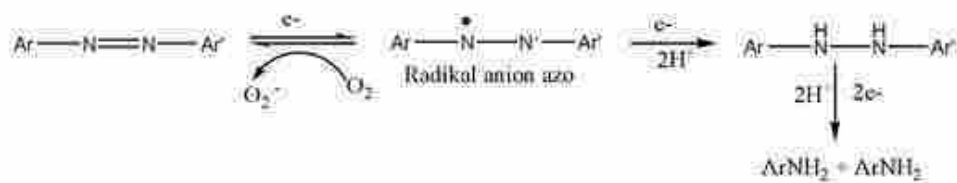
Gambar 29. Reduksi Gugus Azo
