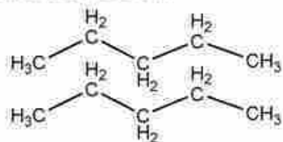
Gambar 9. Interaksi Van der Waals
