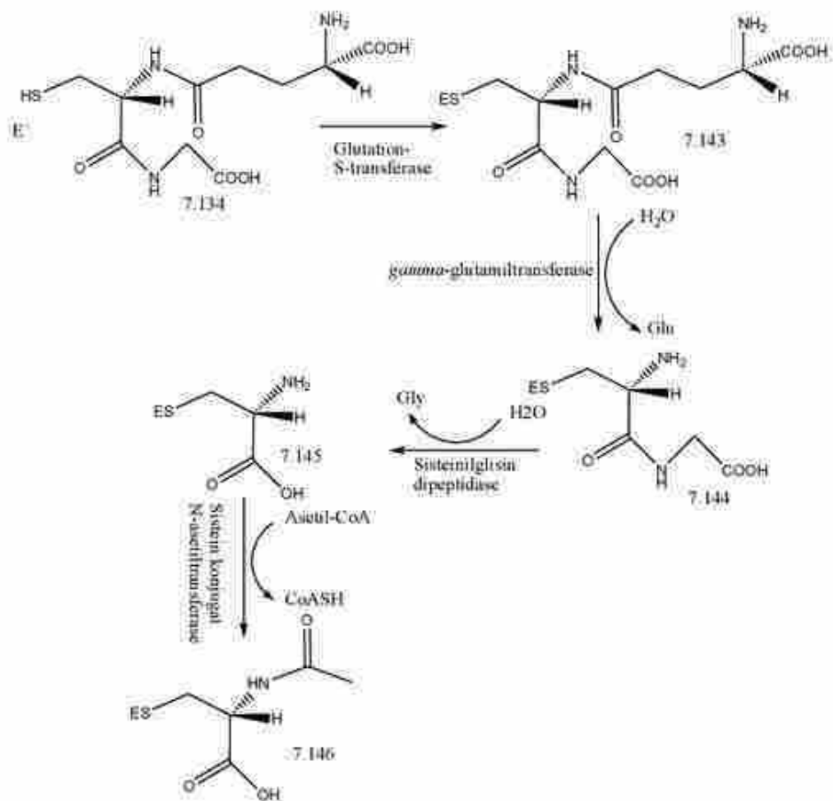
Gambar 38. Metabolisme Konjugat Glutathion menjadi Konjugat Asam Merkapturat
