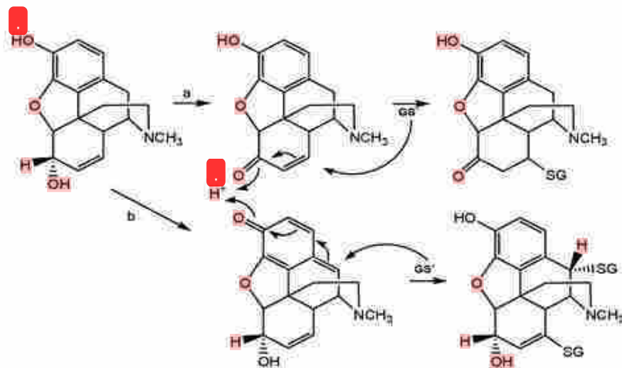
Gambar 39. Contoh Reaksi Konjugasi dengan Glutathion
