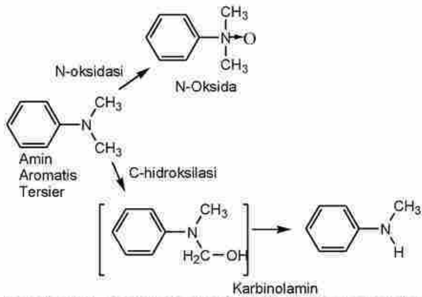
Gambar 58. Biotransformasi Amin Aromatis Tersier
