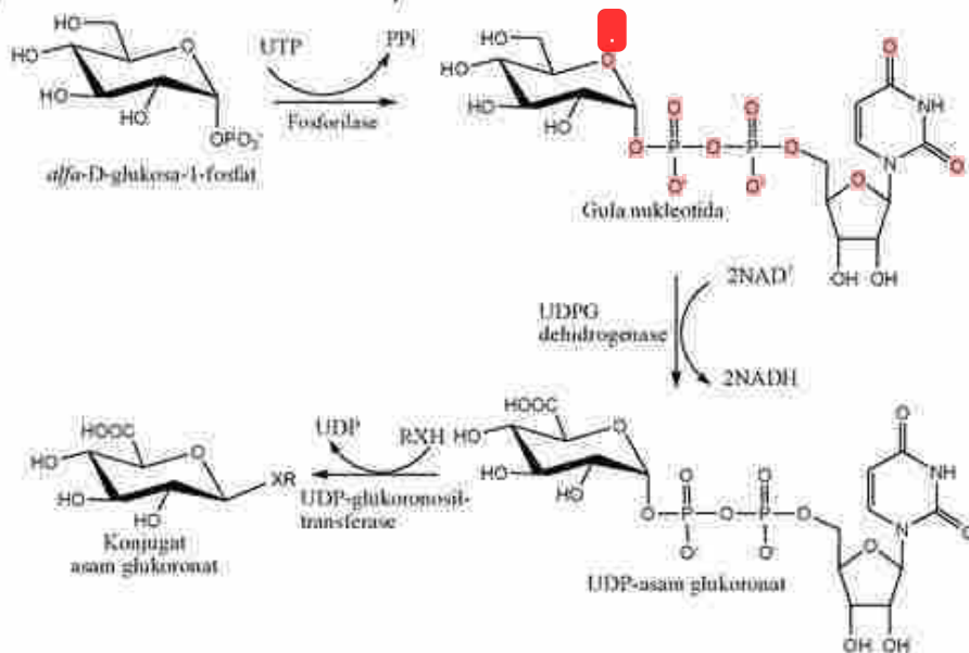
Gambar 33. Jalur Biosintesis dan Reaksi UDP-Asam Glukoronat
