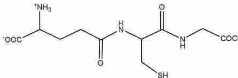
Gambar 37. Struktur Glutathion (GSH)
