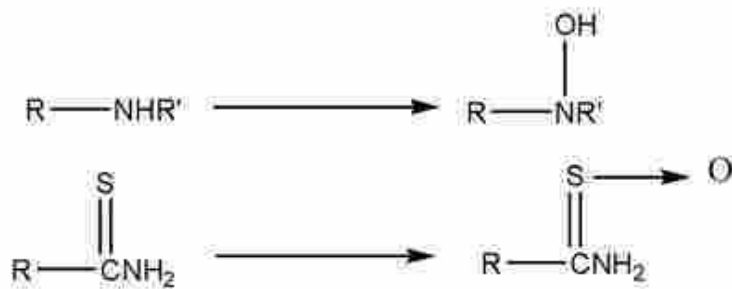
Gambar 22. Substrat untuk Flavin Monooksigenase
