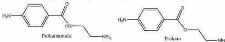
Gambar 25. Hidrolisis Gugus Amida pada Prokainamida menjadi Procain
