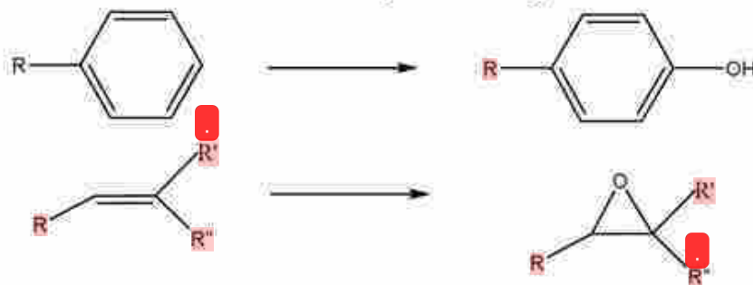
Gambar 21. Substrat untuk Sitokrom P-450
