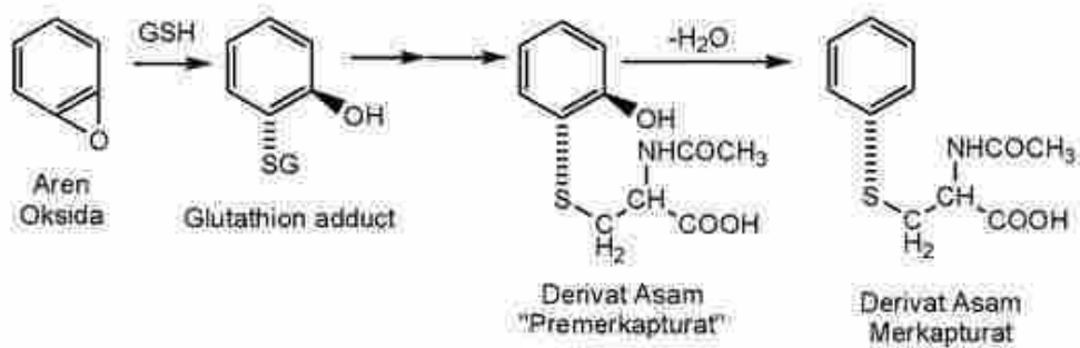
Gambar 46. Biotransformasi Aren Oksida dan Pembentukan Turunan Merkapturat
