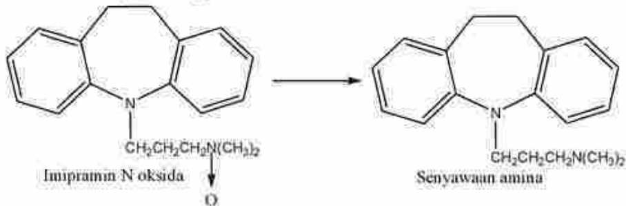
Gambar 31. Reduksi Gugus Amina Oksida Tersier
