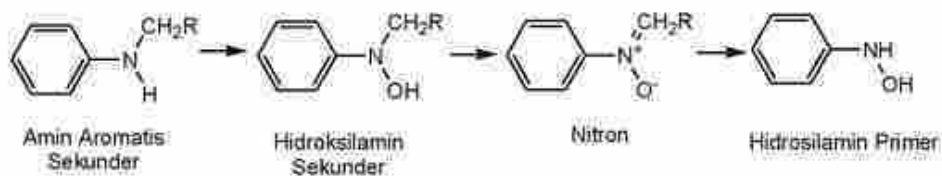
Gambar 59. Biotransformasi Amin Aromatis Sekunder
