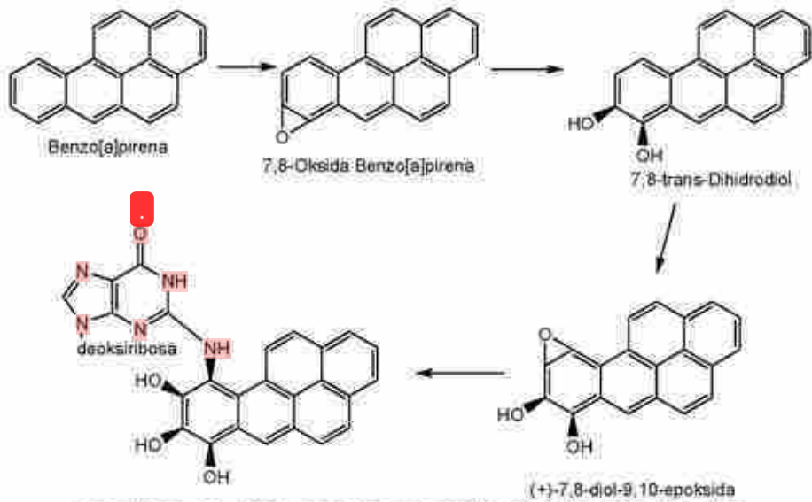
Gambar 44. Biotransformasi Benzo[a]pirena dan Reaksinya dengan Guanosisin
