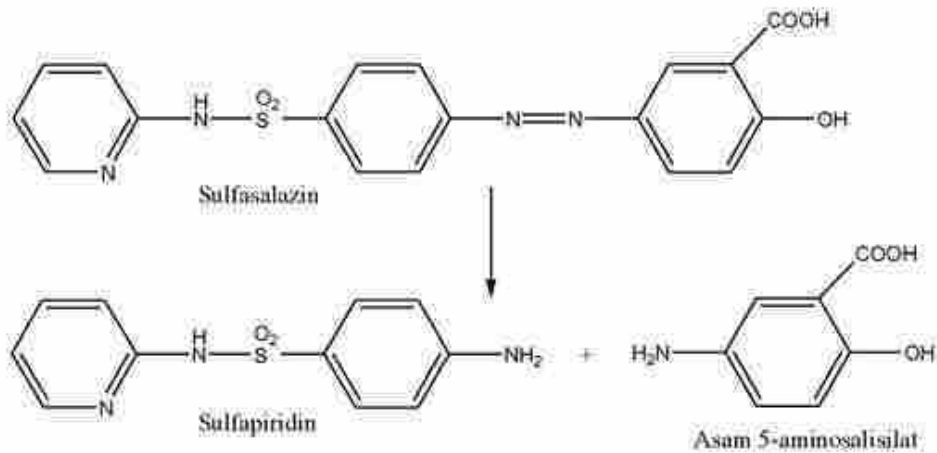
Gambar 30. Metabolisme Reduksi Sulfasalazin
