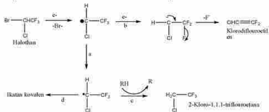
Gambar 32. Reduksi Dehalogenasi Haloethan
