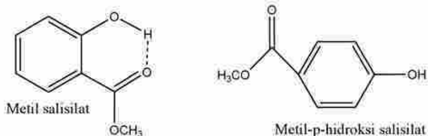
Gambar 4. Metil Salisilat dan Metil-p-Hidroksi Salisilat
