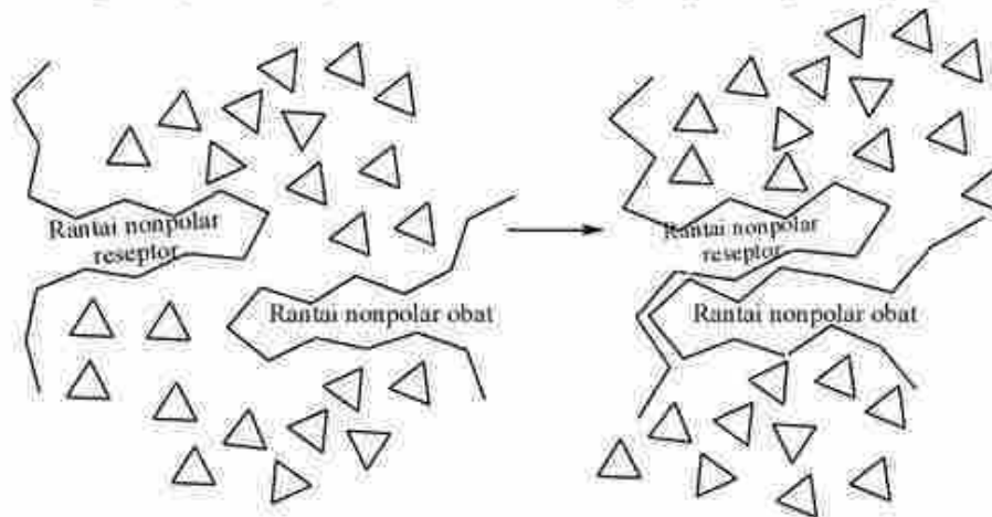
Gambar 7. Pembentukan Interaksi Hidrofobik
