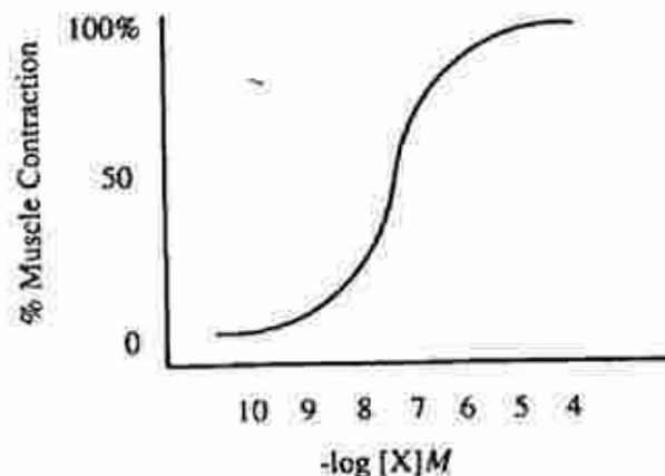
A. Kurva dosis-respon untuk agonis
