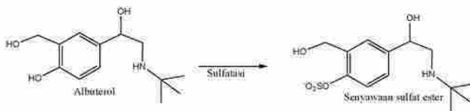
Gambar 34. Reaksi Konjugasi Sulfat pada Albuterol
