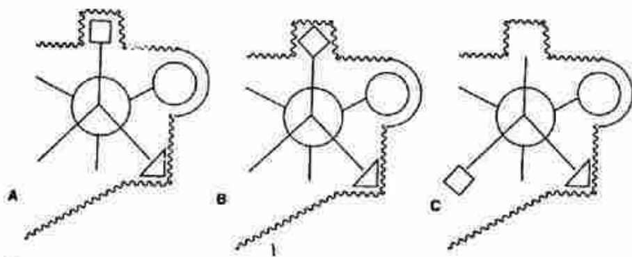
Gambar 13. Interaksi Gugus Obat pada Receptor Binding Site
