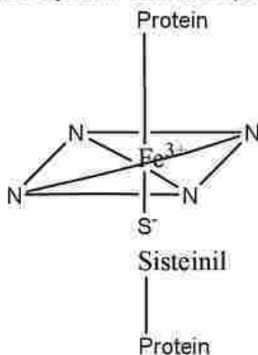
Gambar 17. Kompleks sitokrom P-450
